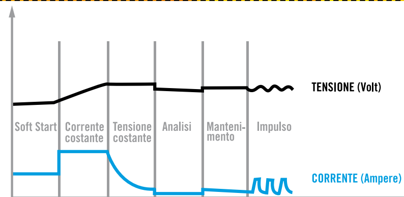
DIAGRAMMA DELLE CARATTERISTICHE DI CARICA
